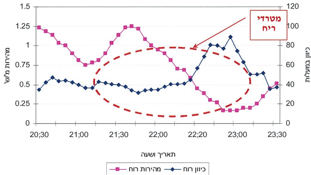
גרף 6: כיוון ומהירות רוח בברקאי בתאריך 6/6/09 - ממוצע רץ 5 דקות
