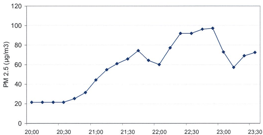
גרף 7: מהלך תקופתי של החלקיקים הנשימים העדינים בתאריך 6/6/09
